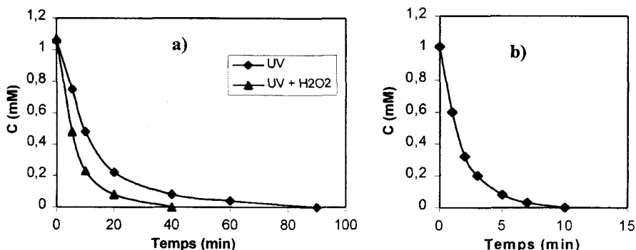
Figure 4 Exemple de courbes cinétiques de dégradation photochimique pour le MCP.
