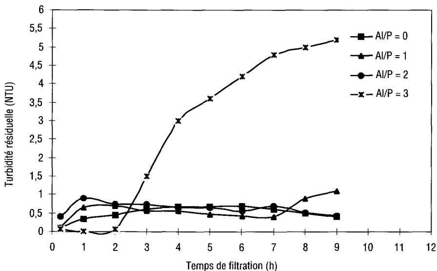
Figure 11 Variation de la turbidité résiduelle en fonction du temps de filtration et du rapport massique Al/P ( V_f = 10 m/h ; G = 50 s -1 ; T_f = 10 mn ; pH = 6,5 ; C_p = 2 mg/l). Variation of residual turbidity turbidity against filtration time and Al/P mass ratios.
