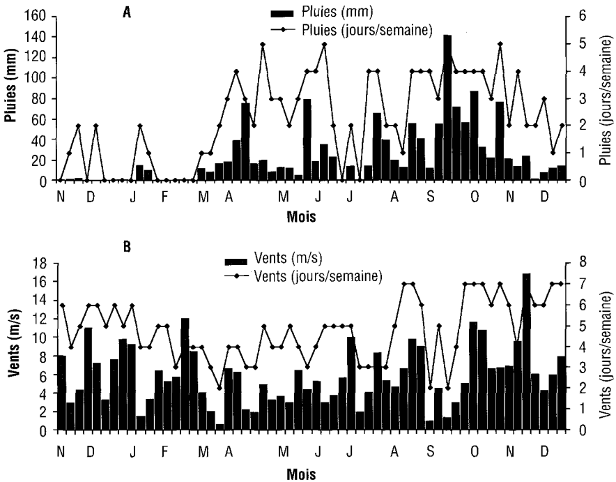
Figure 1 Pluviométrie (A) et régime des vents (B) dans la région de Yaoundé de novembre 1996 à décembre 1997.
