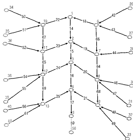
Figure 2 Type de réseau ramifié/maillé appartenant à la classe V ( 60 < D < 80 ). Class V looped/Branched Network ( 60 < D < 80 ).
