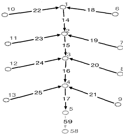
Figure 1 Type de réseau ramifié appartenant à la classe II ( 20 < D < 40 ). Class II Branched Network ( 20 < D < 40 ).
