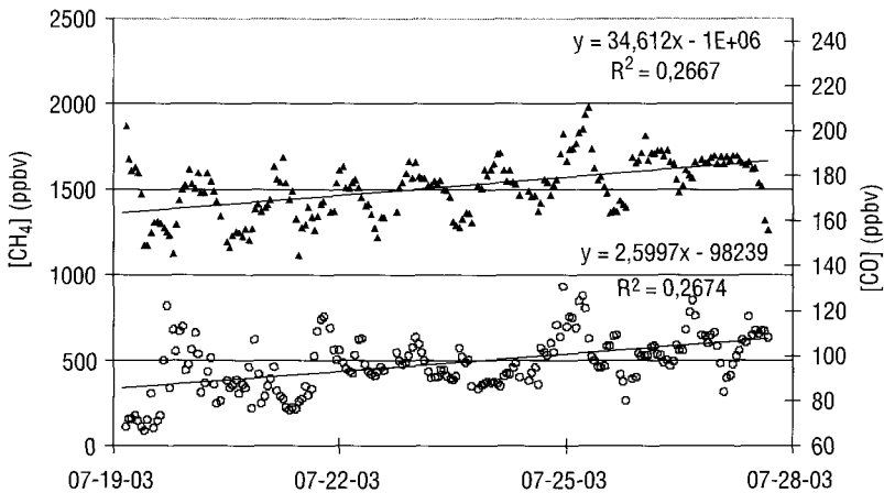
Figure 2 Variations diurnes des concentrations de CH 4 (▲) et de CO (○) troposphériques en fonction du temps. Les courbes de régression linéaires sont illustrées pour montrer l'augmentation du CH 4 et du CO durant cette période. Un long épisode de pluie fut observé entre le 21 et le 27 juillet (33,2 mm de précipitations).
