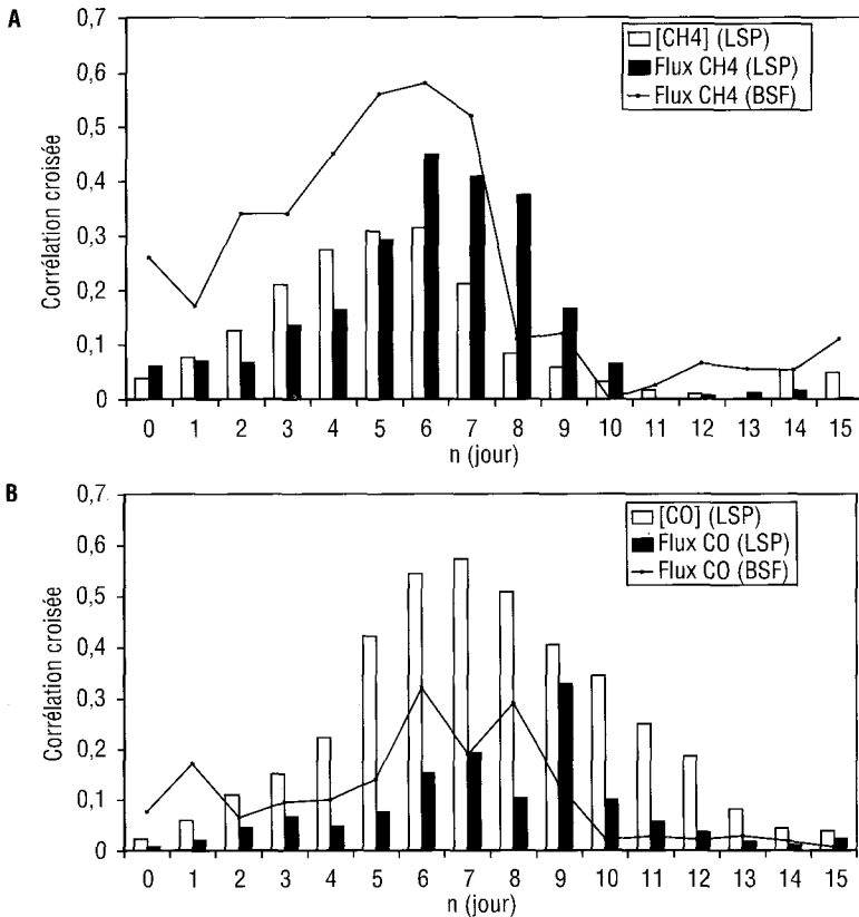
Figure 5 Corrélations croisées entre les concentrations (□) et les flux (■) de (A) CH 4 , (B) CO, (C) H 2 et (D) CO 2 en fonction du niveau du lac Saint-Pierre (LSP) et de la Baie Saint-François (BSF).
