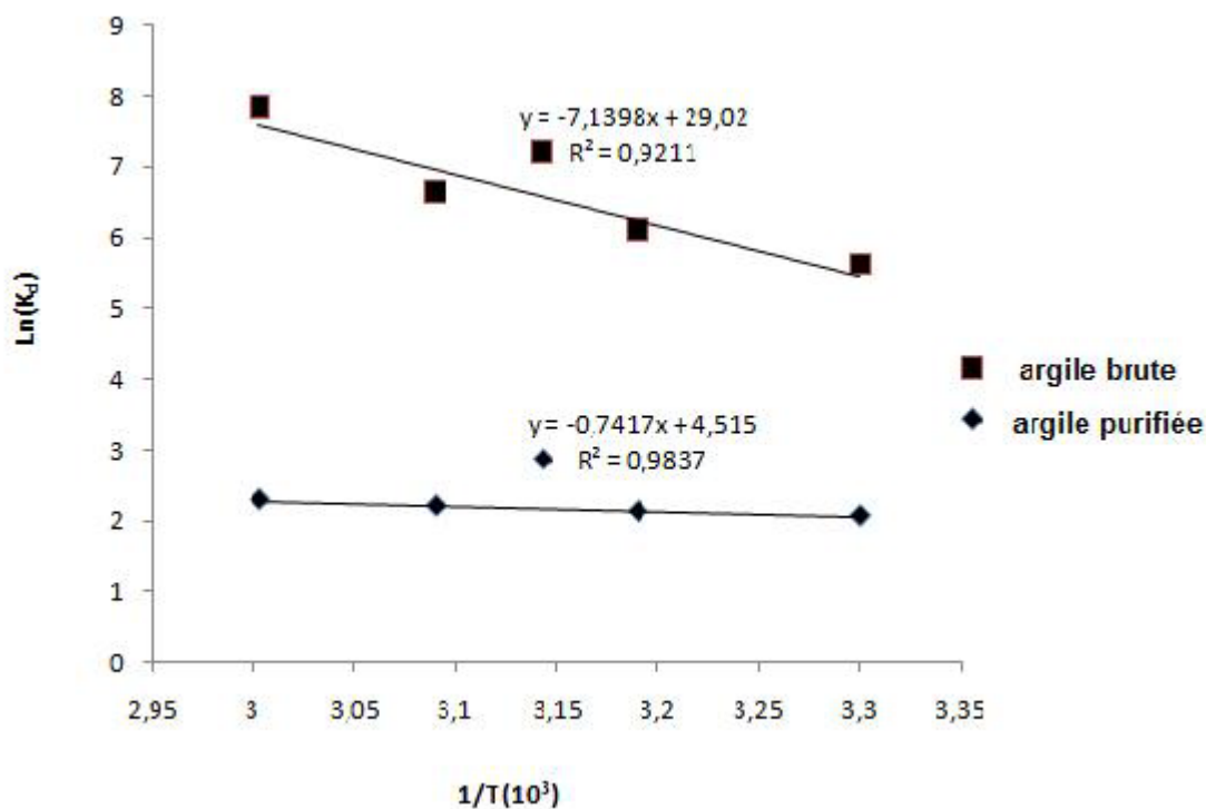
Figure 9. Représentation de \ln(K_d) en fonction de la température ( 1/T ) pour une concentration en colorant de 24 \text{ mg}\cdot\text{L}^{-1} .
