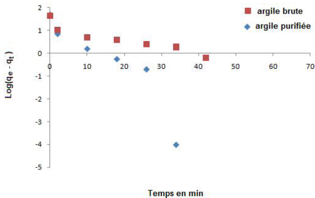
Figure 7. Représentation du modèle cinétique 'pseudo-premier-ordre' pour l'adsorption d'une solution du colorant bleu de méthylène ( 20 \text{ mg}\cdot\text{L}^{-1} ) sur l'argile brute et purifiée.
