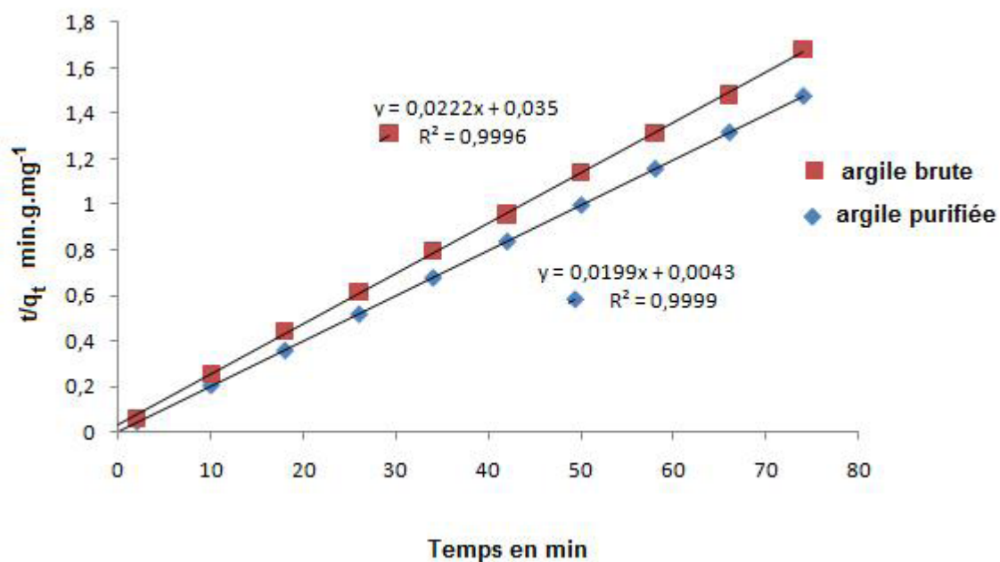
Figure 8. Représentation du modèle cinétique 'pseudo-second-ordre' pour l'adsorption d'une solution du colorant bleu de méthylène ( 20 \text{ mg}\cdot\text{L}^{-1} ) sur l'argile brute et purifiée.
