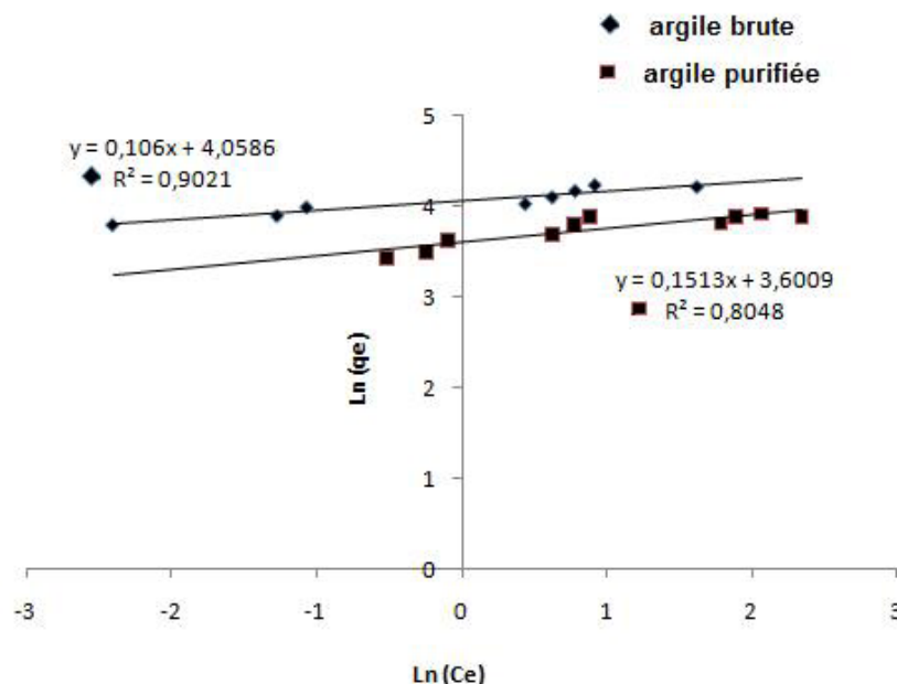
Figure 11. L'isotherme de Freundlich de l'adsorption du bleu de méthylène sur l'argile brute (◆) et l'argile purifiée (■). Freundlich isotherm for the adsorption of methylene blue on purified clay (◆) and crude clay (■).
