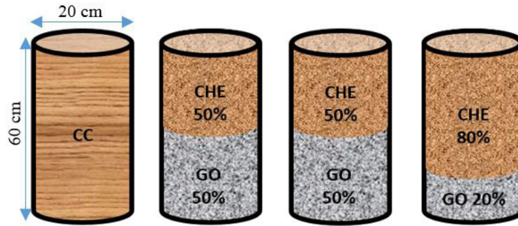
Figure 1. Pilotes de biofiltration : CC : copeaux de coco; CHE : chènevotte; GO : grignons d'olives. Biofiltration pilots: CC: coconut husks; CHE: hemp shives; GO: olive pomace.
