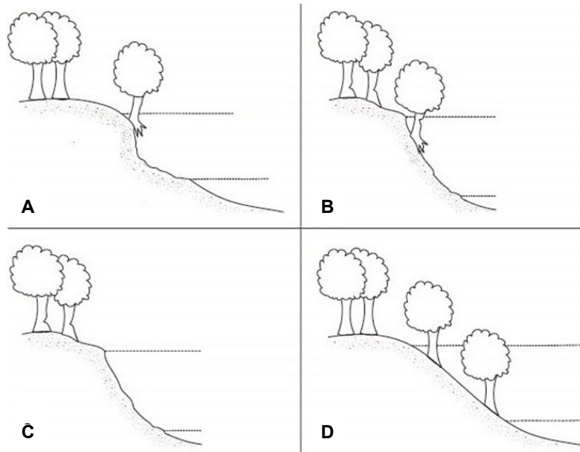
Figure 3. Morphotypes de berges résultant du classement par dendrogramme : A) berges d'érosion fluviale, B) berges glacielle - érosion modérée, C) berges glacielles - érosion forte, D) berges stables ou en accrétion. Les lignes représentent la division visuelle de la berge en trois parties effectuée lors de la collecte de données.
