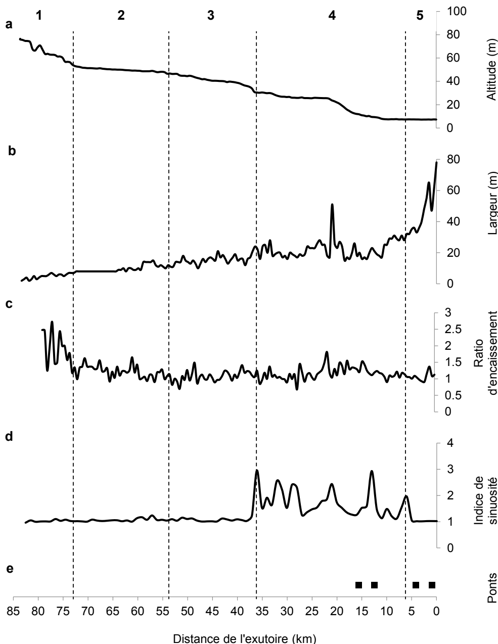
Figure 2. Caractérisation du chenal selon divers indicateurs morphométriques. Les lignes pointillées délimitent les différents secteurs homogènes à l'étude. Channel characterization according to several morphometric indicators. Dotted lines represent homogenous sectors.
