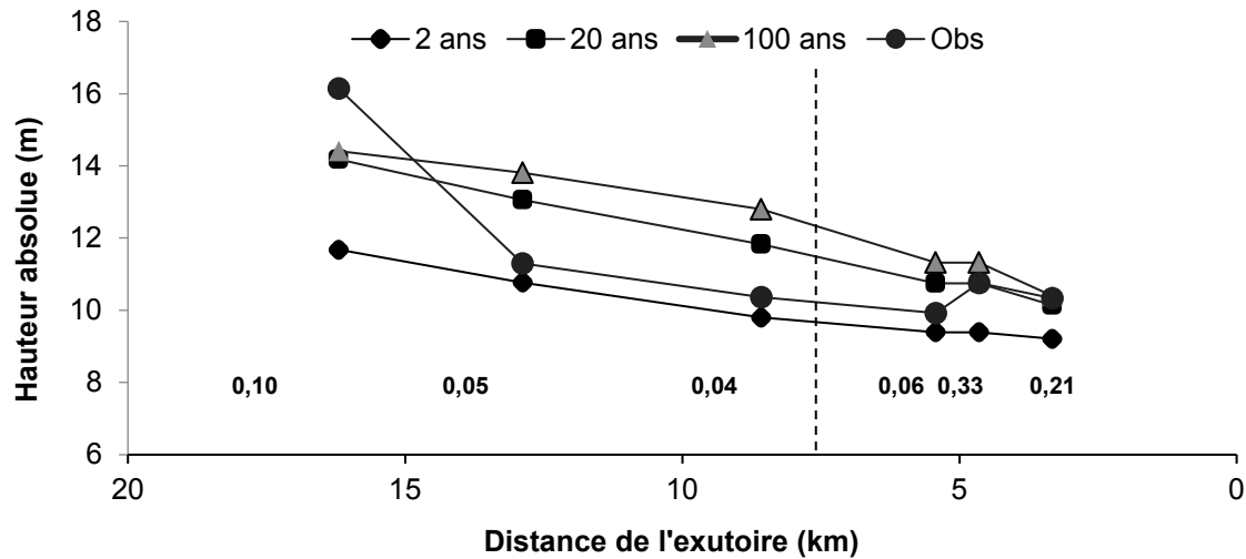
Figure 7. Comparaison entre les hauteurs absolues des cicatrices glacielles (en mètres) et les cotes de crues du Programme de détermination des cotes de crue (PDCC). La ligne pointillée représente la séparation entre les secteurs 4 et 5 et les nombres en gras la fréquence des événements observés sur le terrain par site.
