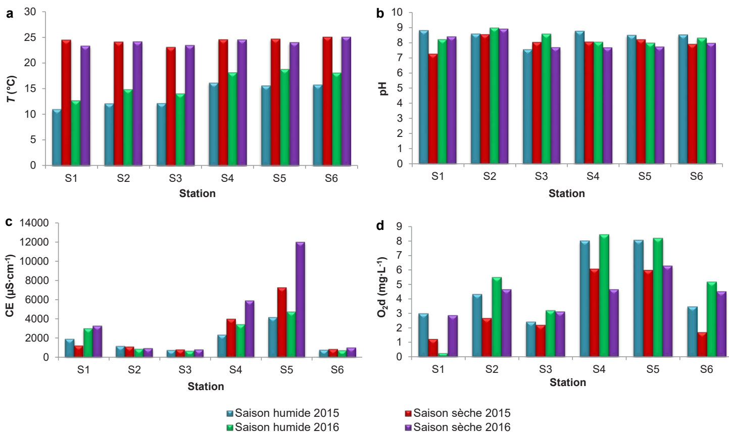
Figure 3. Variation des paramètres physicochimiques des eaux superficielles du lac Fetzara : a) température ( T ), b) pH, c) conductivité électrique (CE), d) oxygène dissous ( O_2d ). Variation in the physico-chemical parameters of the surface waters of Lake Fetzara: a) temperature ( T ), b) pH, c) electrical conductivity (EC), d) dissolved oxygen ( O_2d ).
