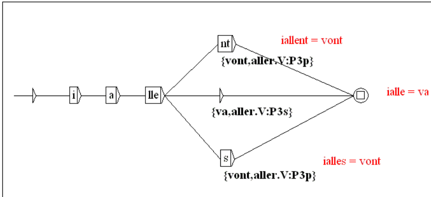
Figure 4 : Transducteur des différentes formes graphiques du verbe aller en français acadien
