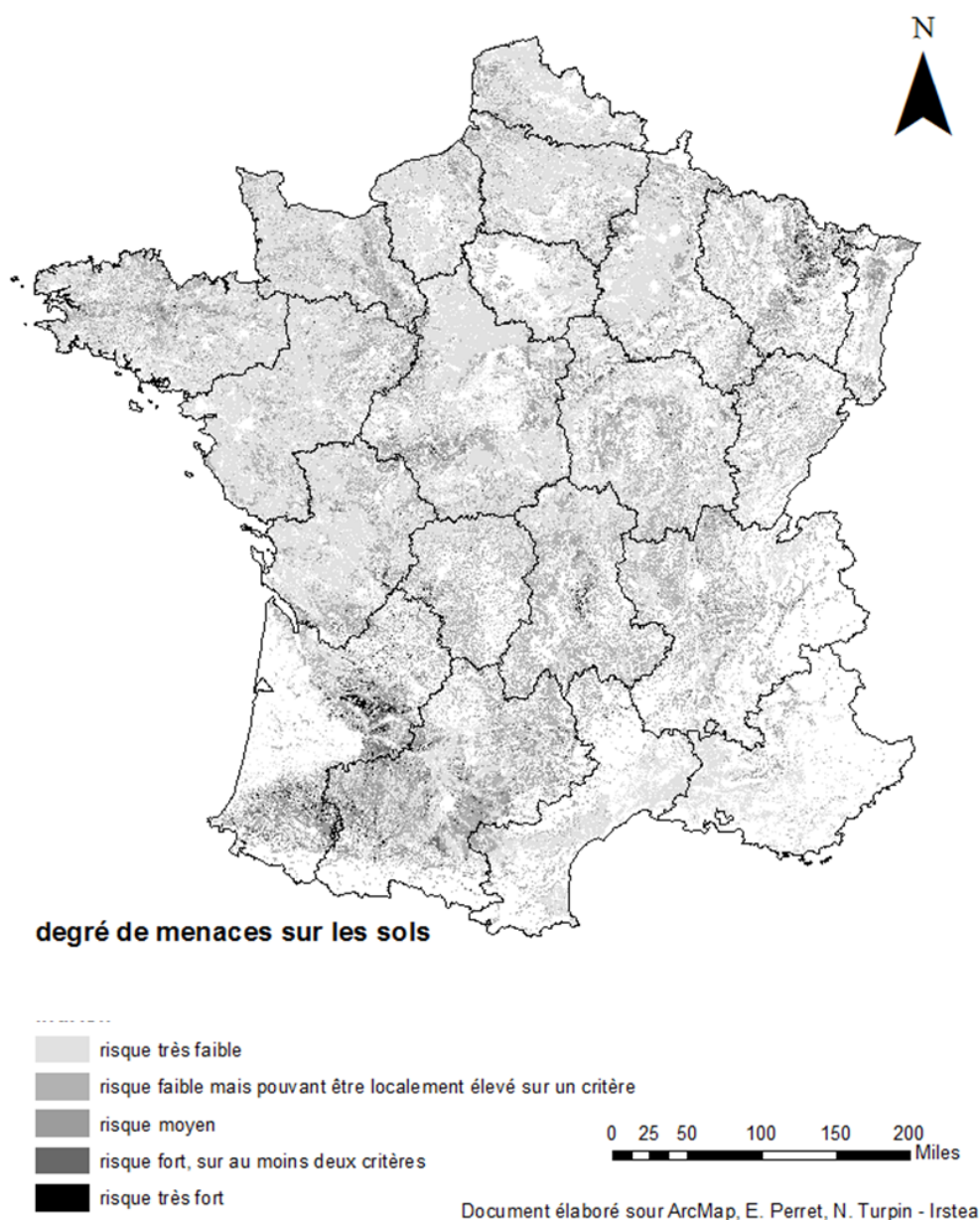
Figure 1. Degré de menaces sur les sols.
