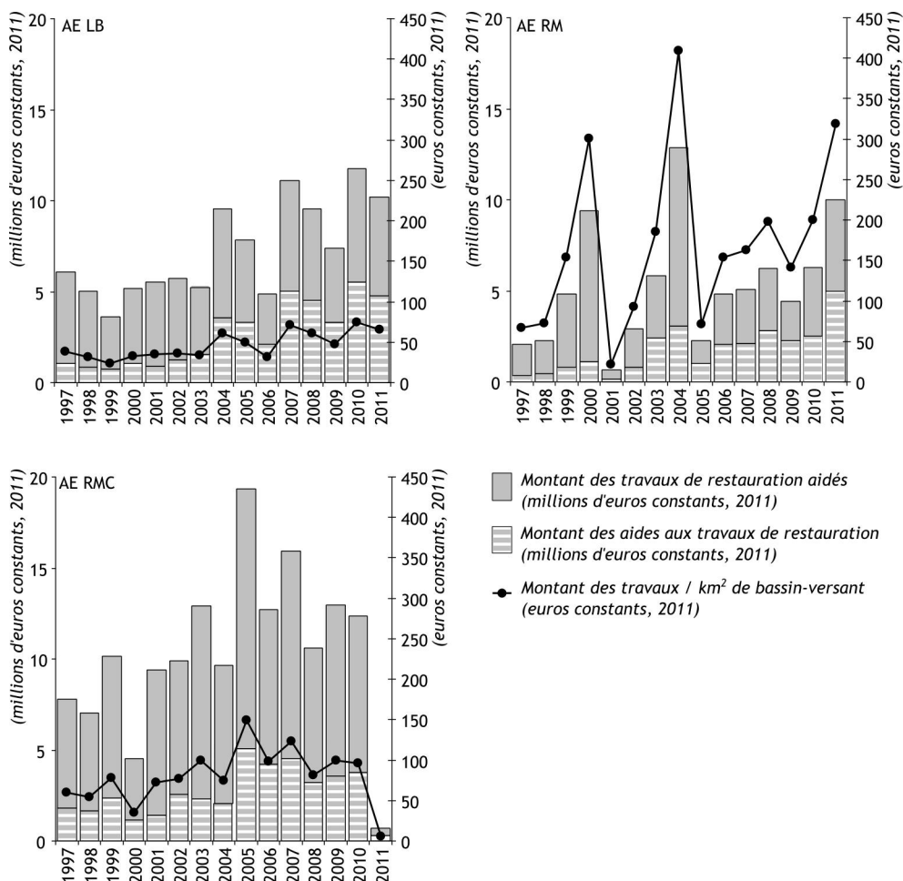
Figure 5. Les volumes financiers des dossiers d'aides instruits par les AE LB, RM et RMC (1997-2011) en montant absolu et en montant relatif à la taille des différents bassins-versants.
