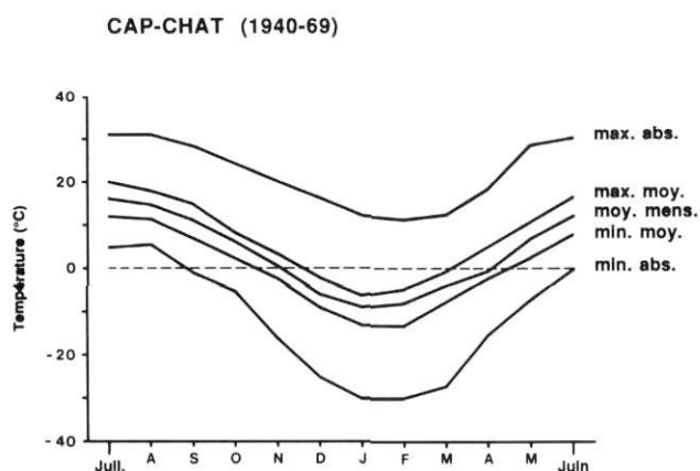
FIGURE 5. Le régime des températures dans le nord de la Gaspésie (station de référence: Cap-Chat). De haut en bas: les températures maximales absolues, les températures maximales moyennes, les moyennes mensuelles, les températures minimales moyennes, les températures minimales absolues.
