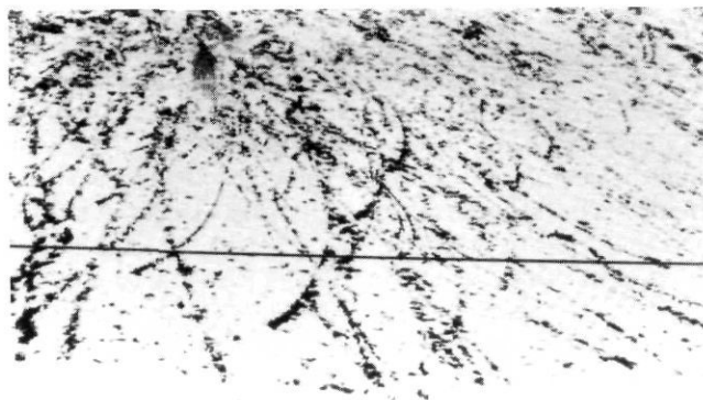
FIGURE 22. Talus T-2, 20 mars 1980. Traces de pierres roulées sur une neige tardive, très mince (neige mouillée).
