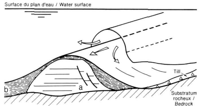
FIGURE 6. Construction d'un esker « rétrogressif » dans un lac proglaciaire à l'embouchure d'un tunnel sous-glaciaire : (a) sédiments mis en place dans le tunnel, (b) sédiments proglaciaires d'épandage (simplifié de Sharpe, 1988).
