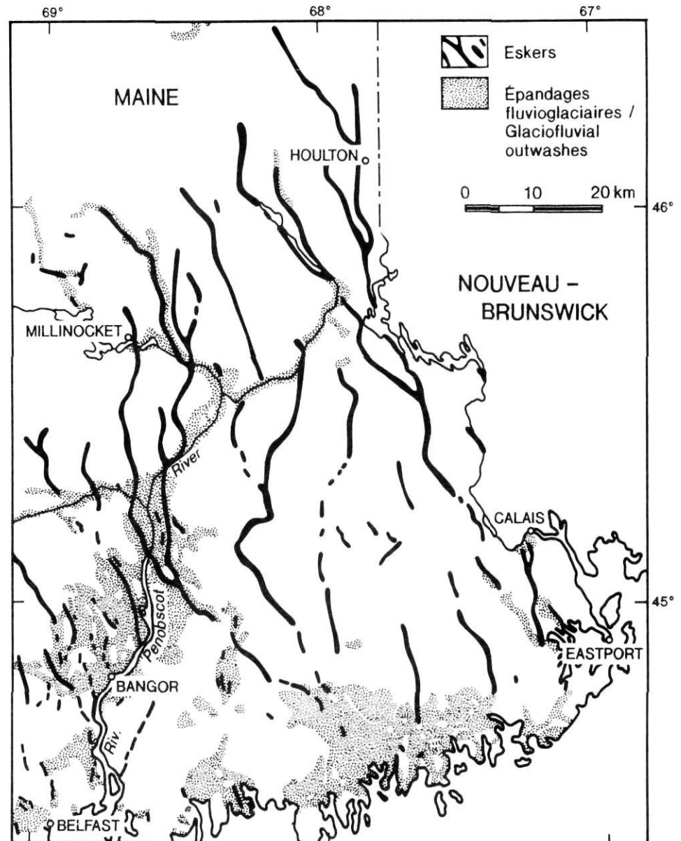
FIGURE 3. Distribution des eskers et des épanchages fluvioglaciaires dans l'état du Maine, États-Unis (source : Charlesworth, 1957).
