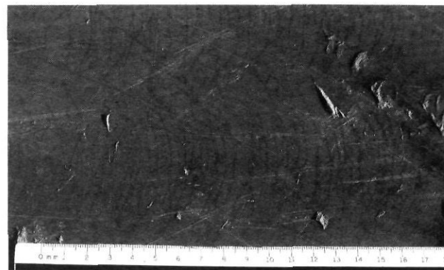
FIGURE 3. Fractures de broutage virtuelles soulignées par la coloration foncée de la roche dolomitique (écoulement des glaces vers la gauche), Saint-Eustache, Québec.
