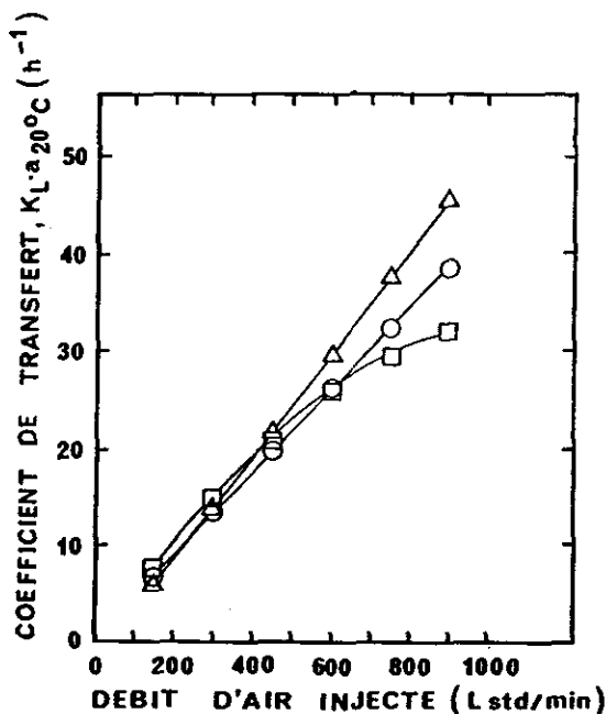
Figure 8.- Variation du coefficient global de transfert d'oxygène ( K_L.a_{20°C} ) en fonction du débit d'air total injecté pour l'injecteur poreux ( \Delta ), l'aérateur à cheminement prolongé ( \square : répartition proportionnelle) et le système hybride ( \circ : répartition proportionnelle).
