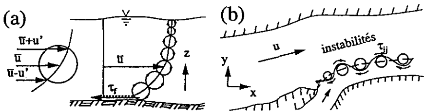
Figure 4 Macro-structures turbulentes dans un écoulement fluvial.
