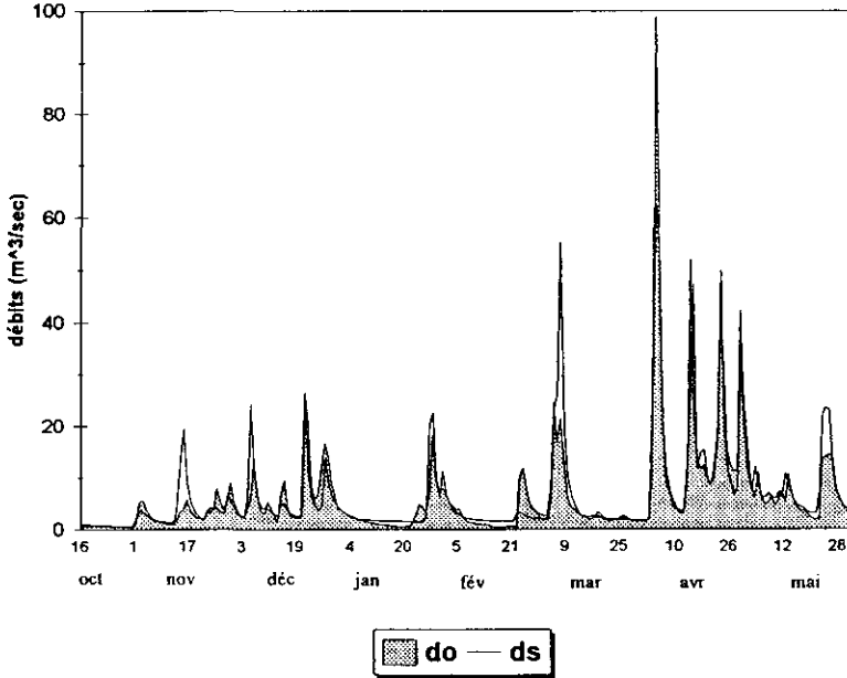
Figure 3a Simulations des débits à la station 030242 sur le bassin de la rivière Clifton, au Québec.
