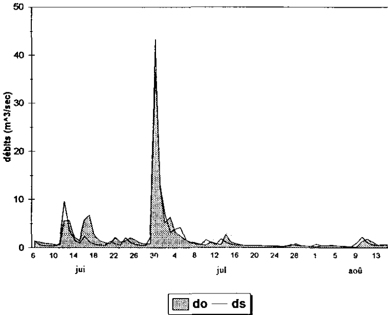
Figure 3b Simulations des débits à la station 030242 sur le bassin de la rivière Clifton, au Québec. Streamflow simulations at station 030242, on the Clifton river in Québec.
