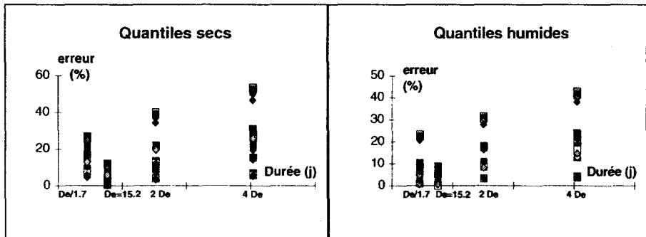
Figure 27 Bassin versant de l'Allier à MONISTROL d'ALLIER ( S = 988 \text{ km}^2 ). Allier's basin at MONISTROL D'ALLIER ( S = 988 \text{ km}^2 ).
