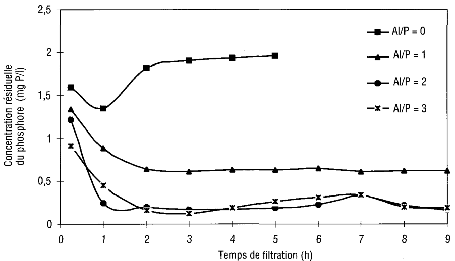
Figure 3 Variation de la concentration résiduelle du phosphore en fonction du temps de filtration et du rapport massique Al/P ( V_f = 5 m/h ; T_f = 10 min ; pH = 6,5 ; C_p = 2 mg/l ; G = 50 s ^{-1} ). Variation of phosphorus residual concentration against filtration time and Al/P mass ratios.
