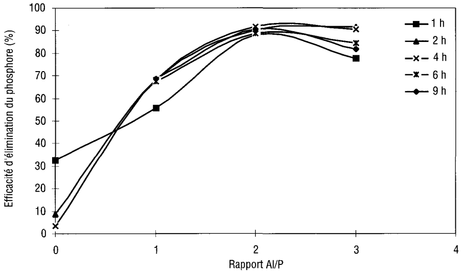
Figure 2 Efficacité d'élimination du phosphore en fonction du rapport massique Al/P ( V_f = 5 m/h ; T_f = 10 min ; pH = 6,5 ; C_p = 2 mg/l ; G = 50 s ^{-1} ). Efficiency of phosphorus removal against Al/P mass ratios.
