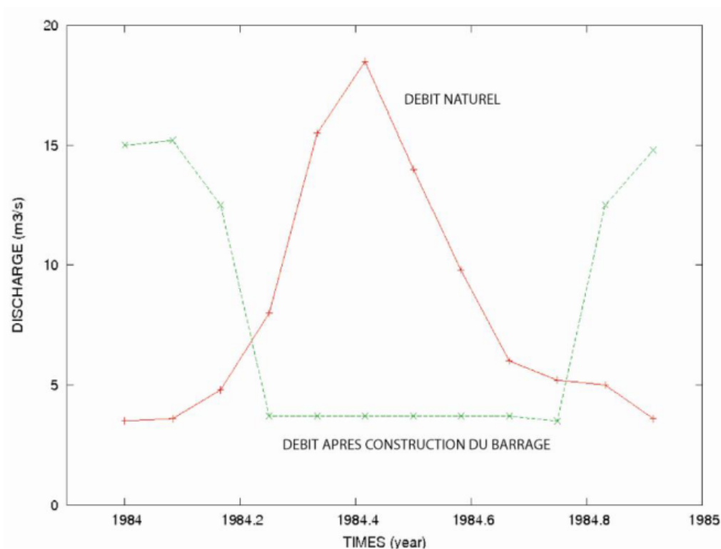
Figure 5. Débit en 1984 de l'Eau d'Olle à La Pernière (Allemont, Isère) avant et après la construction de la retenue de Grand-Maison / Water discharge of the Eau Dolle River in 1984 at La Pernière (Allemont, Isère, French Alps) before and after the construction Grand-Maison Dam
