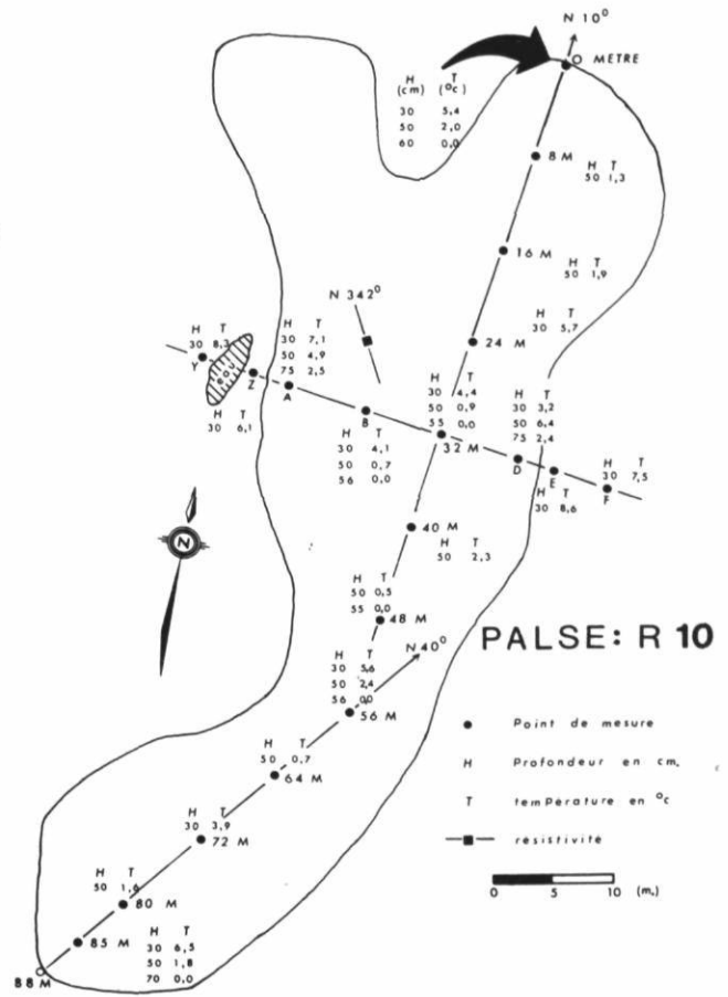
FIGURE 4. Profils thermiques de la palsa n° R-10. Thermal profiles of palsa No. R-10.
