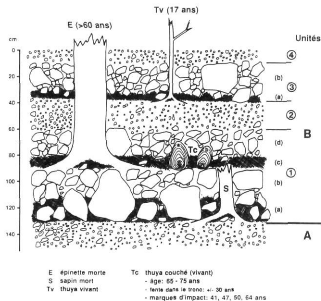
FIGURE 14. Description de la coupe n° 2. Niveaux 1 et 3: lits de blocs roulés; unité A et niveaux 2 et 4: dépôts d'avalanches (graviers); 1a, 1c et 3a: horizons organiques fossiles.
