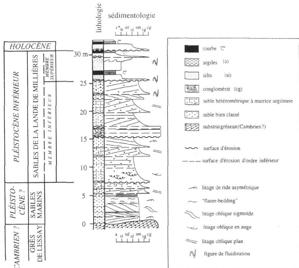
FIGURE 6. Coupe stratigraphique synthétique de la série de La Lande de Millières. τ : tourbe. a : argile. si : silt ; stf : sable très fin. sf : sable fin. sm : sable moyen. sg : sable grossier. cg : conglomérat.
