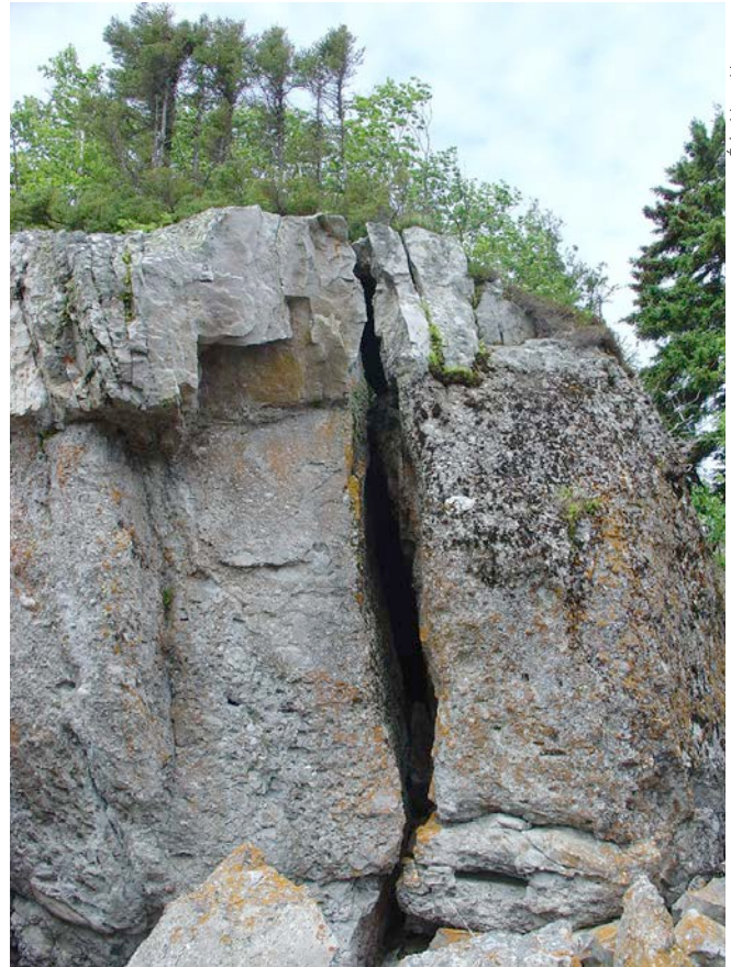
Conglomérats calcaires observés dans la partie nord-est de l'île Dumais.
