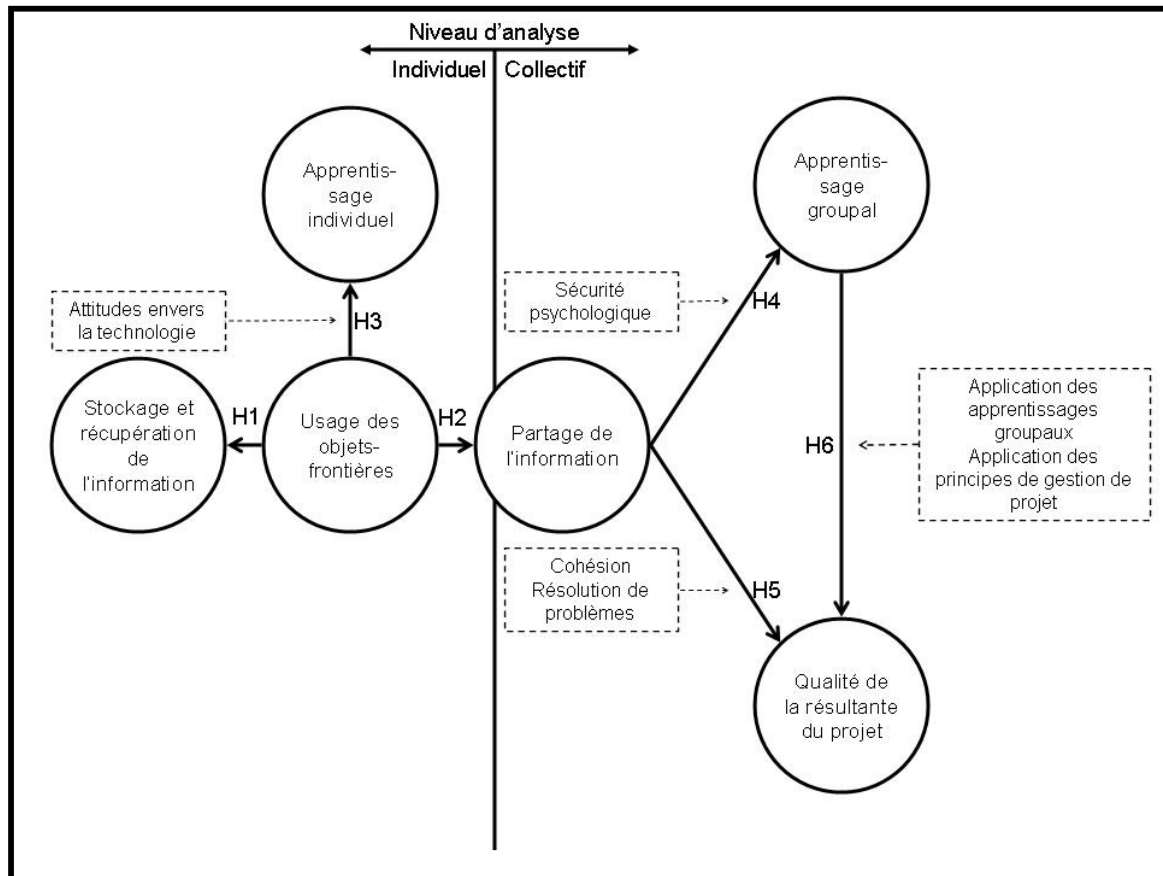
Figure 1. Réseau nomologique
