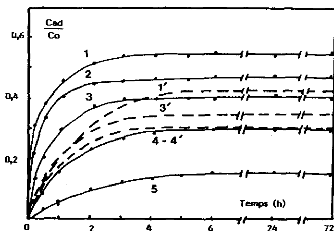
Figure 2 Influence du DSS sur la cinétique d'adsorption des AH ( 10 \text{ mg.l}^{-1} ) sur CAP ( 0,5 \text{ g.l}^{-1} ).
