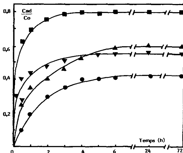
Figure 1 Influence du pH sur la cinétique d'adsorption des AH ( 10 \text{ mg.l}^{-1} ) sur CAP.
