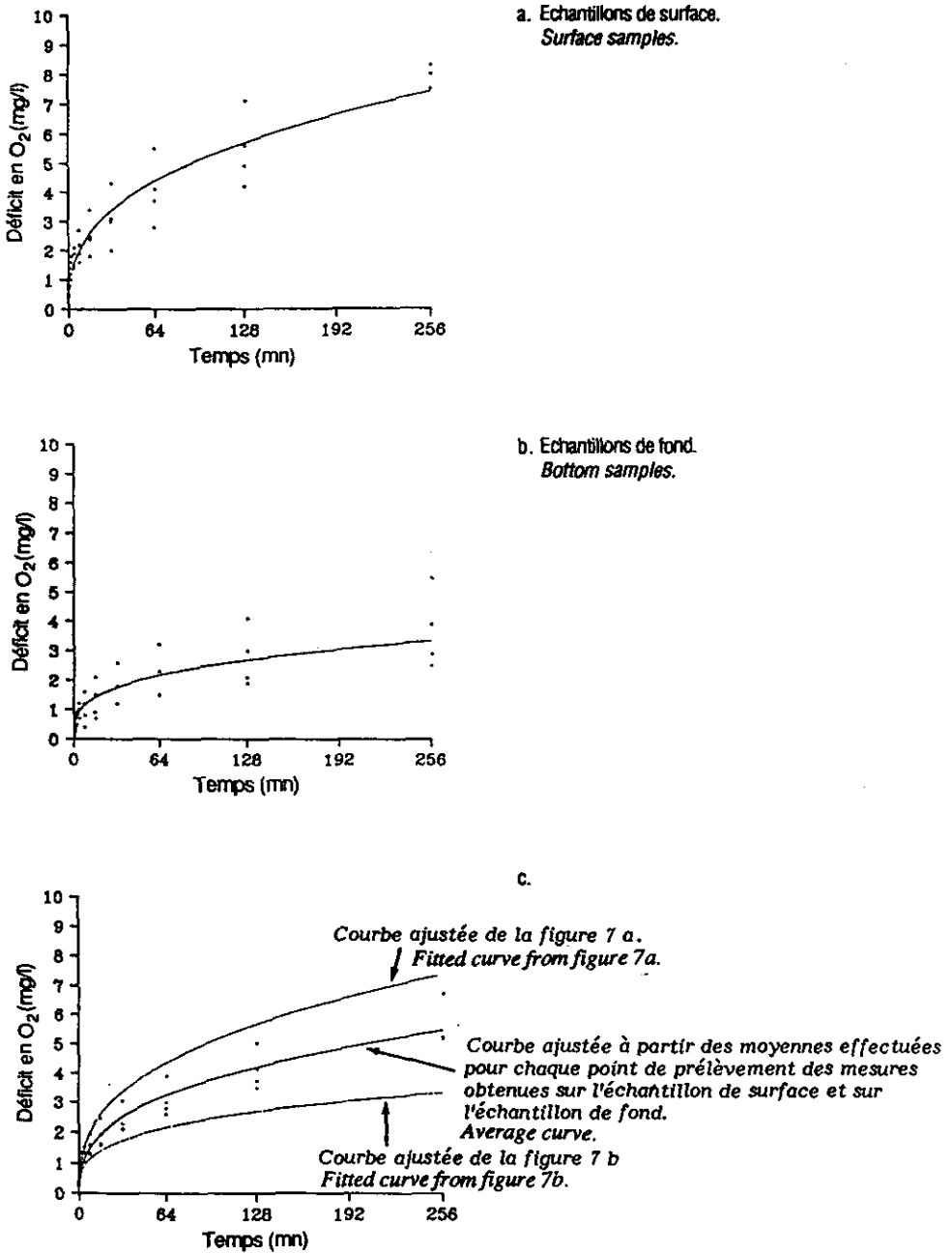
Figure 7 Consommation en oxygène dissous des sédiments de la retenue de Saint-Hilaire (concentration des MES : 5 g/l). Dissolved oxygen consumption of sediments from Saint-Hilaire dam (suspended solids concentration : 5 g/l).
