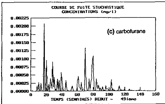
Figure 2 Courbes de fuite stochastique (arrivée à la nappe) calculées par VULPEST pour les pesticides aldicarbe (a), atrazine (b) et carbofurane (c). Breakthrough curves (concentrations reaching the water table) calculated by VULPEST for the aldicarb (a), atrazine (b) and carbofuran (c) pesticides.
