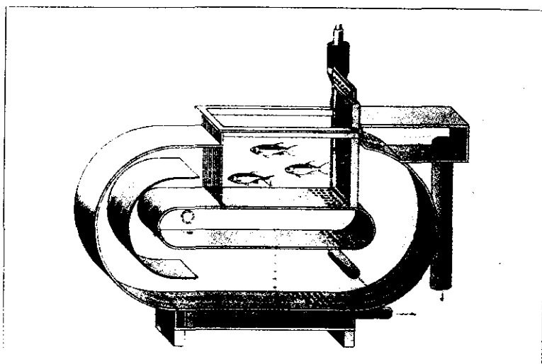
Figure 2 Principe général des biocapteurs basés sur l'étude du rhéotactisme des poissons (d'après BOTTERWEG et al. , 1989).
