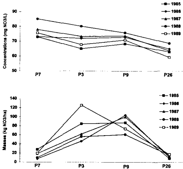
Figure 4 Évolution amont-aval des concentrations mesurées dans la nappe et des flux annuels de nitrates lessivés de la zone non saturée. Upstream/downstream evolution of observed concentrations in the aquifer and calculated nitrate fluxes from the vadose zone.
