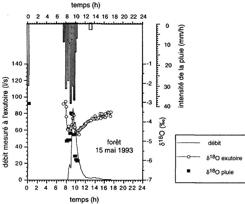
Figure 5 Hydrogramme, hyétogramme (crue du 15 mai 1993, bassin forestier) et évolution temporelle des teneurs en ^{18}O mesurées dans les précipitations et dans l'eau prélevée à l'exutoire du bassin.
