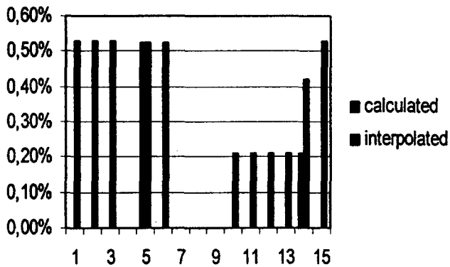
Figure 7 Écarts de hauteurs d'eau sur le réseau de Lyon avec BSV. BSV depth deviations in the Lyon network.
