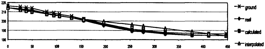
Figure 2 Profil en long du réseau de Lyon. Lyon network longitudinal profile.
