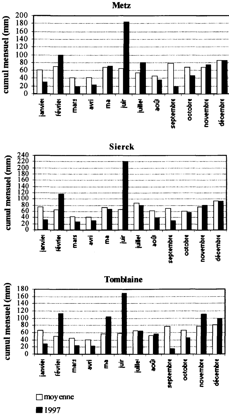
Figure 3 Pluviométrie mensuelle moyenne et en 1997 pour 3 stations météorologiques lorraines.
