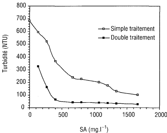
Figure 4 Évolution de la turbidité résiduelle en fonction de la dose de SA ajouté pour un simple traitement et un double traitement à pH 7.
