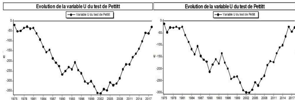
Figure 6. Recherche de rupture sur les débits annuels à la station de Gonsé (Test de Pettitt)
