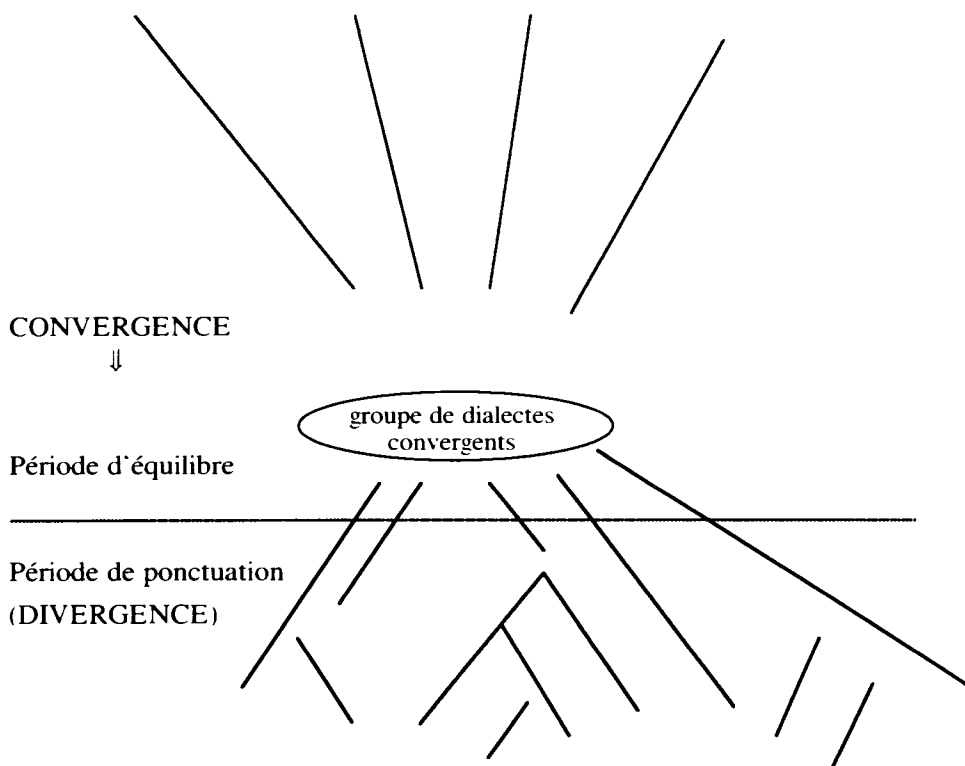
Figure 2 Modèle de l'équilibre ponctué de Dixon
