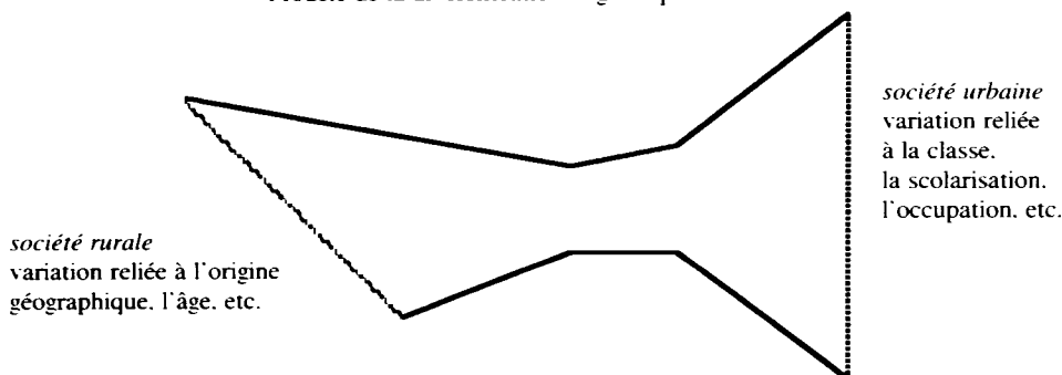
Figure 3 Modèle de la diversification linguistique de Jourdan
