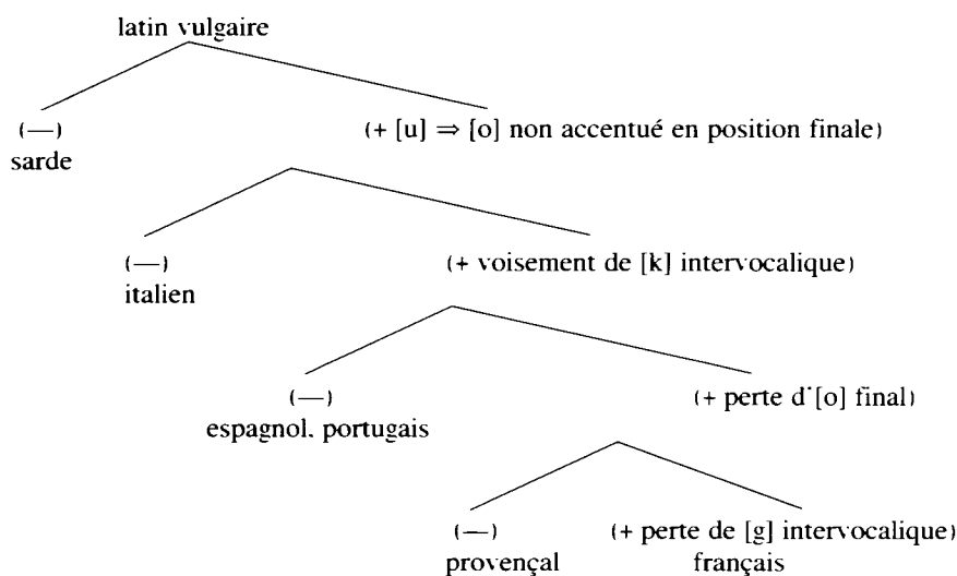
Figure 1 Esquisse d'un arbre généalogique des langues romanes
