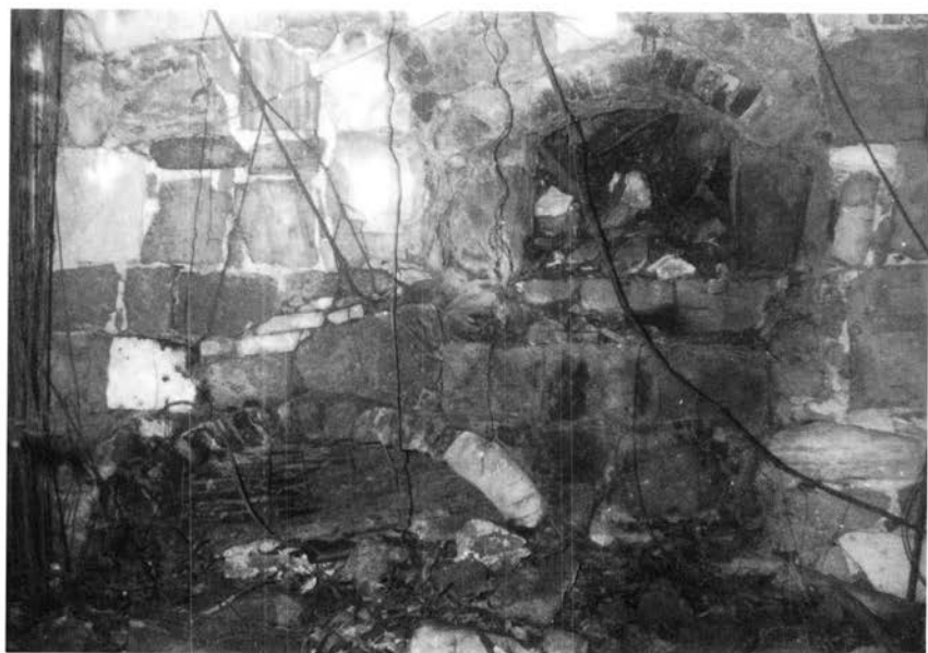
Fig. 12. – Sucrierie : foyer et cendrier de l'équipage.
