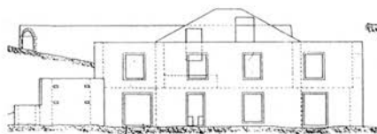
Facade Sud (bâiment 3 et portique 11 étendu)
