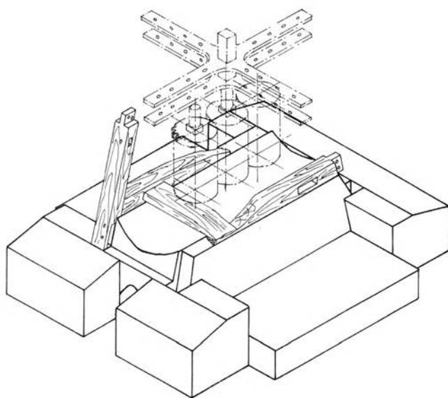
Habitation SPRING Moulin : socle du mécanisme, position probable des rôles.
