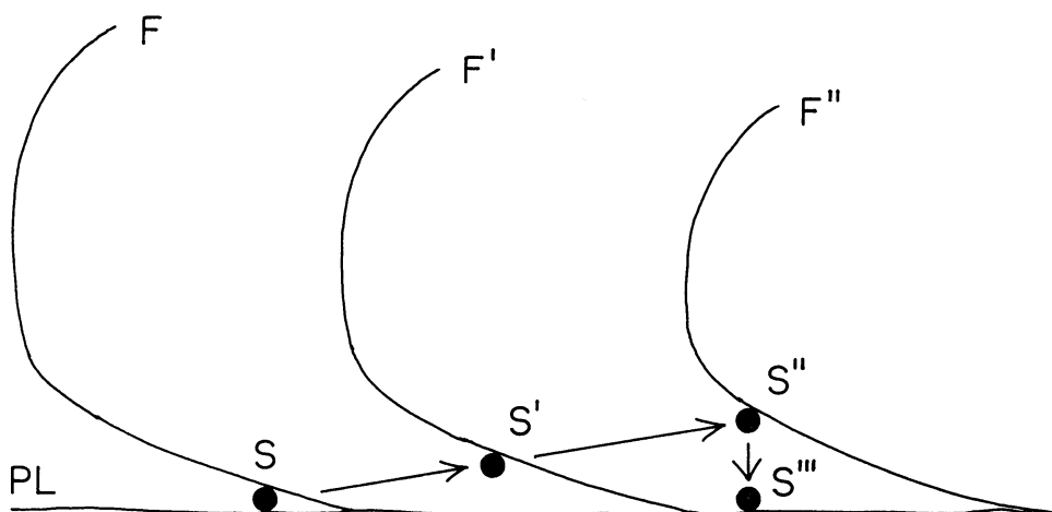
Figure 1 Vue en coupe des positions successives d'une particule de sable S, prise en charge par un bloc de glace en fusion, de F à F'', qui quitte en S' la surface de la plage PL, et se retrouve enfin de course en S'' à la périphérie du bloc; jointe à d'autres grains sablonneux au cours du cheminement, la particule se détache du plafond et se retrouve en S''' sur le plancher de la plage.
