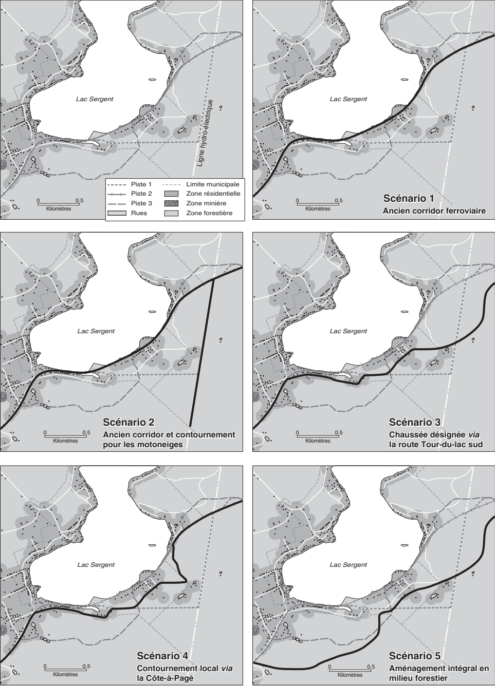
Figure 3 Projet de piste cyclable. Scénarios d'aménagement des cinq meilleurs tracés. Municipalité de Lac-Sergent, MRC de Portneuf, 1996
