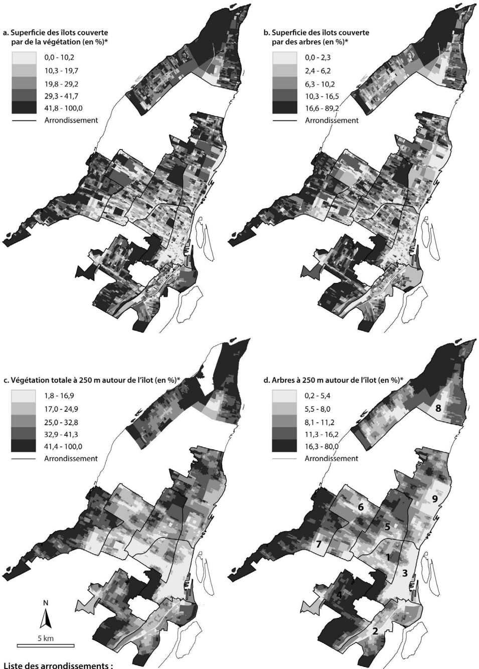
Figure 1 Cartographie de quelques indicateurs de végétation
