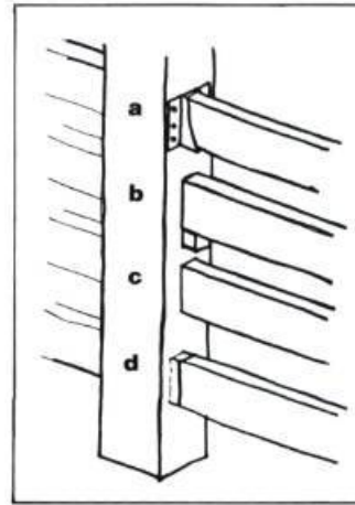
Les façons d'assembler les traverses aux poteaux:
