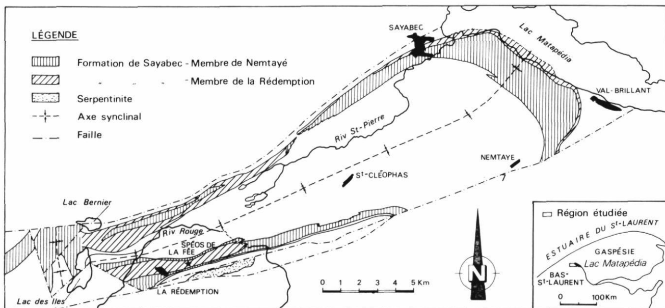
FIGURE 1. La formation de Sabayec dans le synclinal du lac Matapédia, simplifié d'après HÉROUX (1975).
