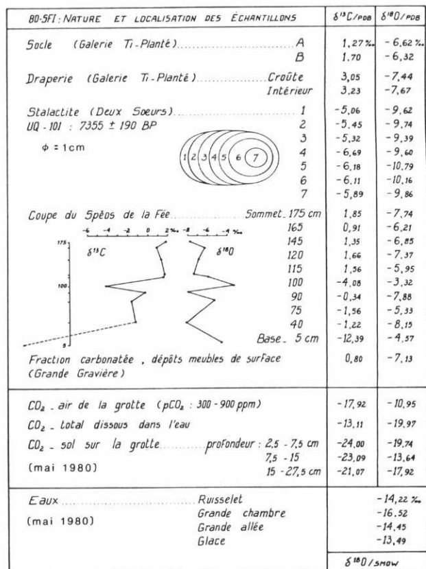
FIGURE 6. Composition isotopique de \text{CO}_2 , de l'eau et des carbonates du Spéos de la Fée.
