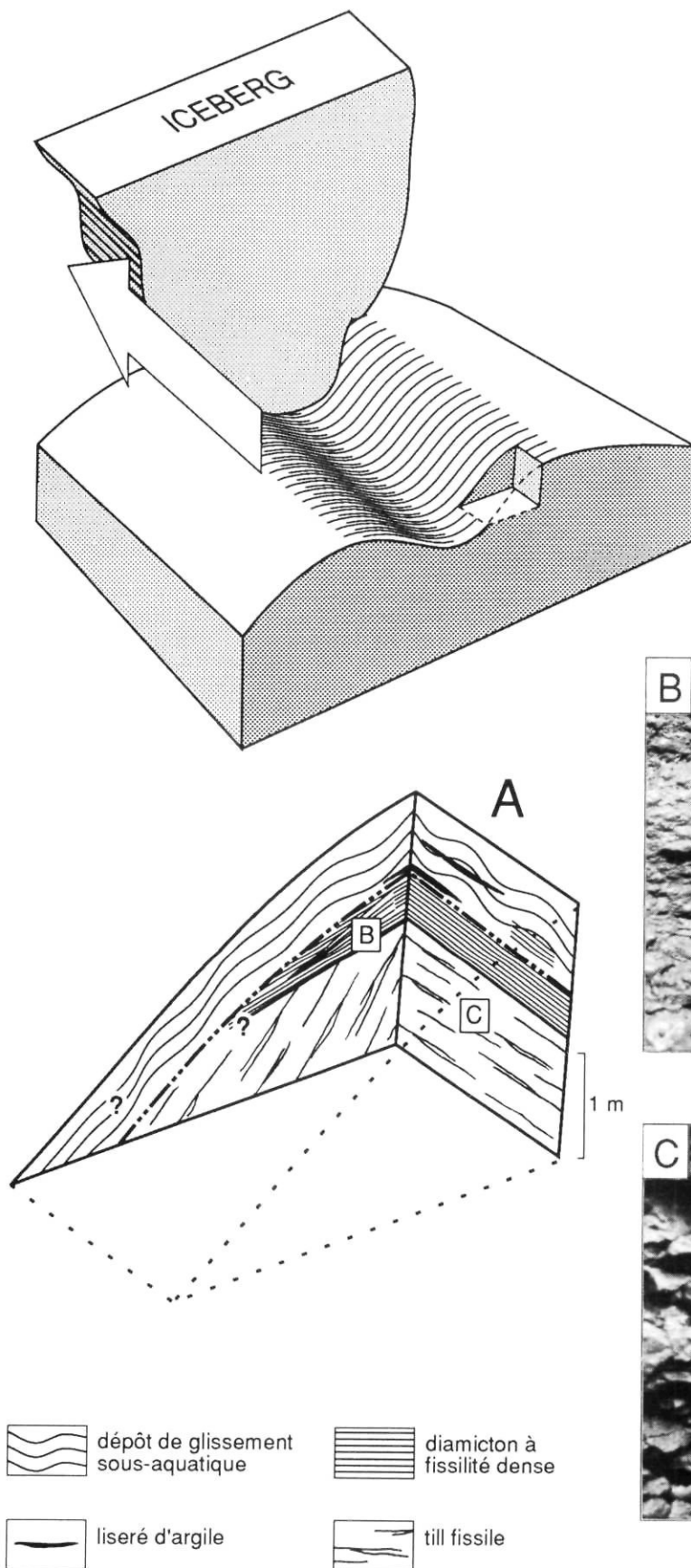
FIGURE 7. La coupe ouverte dans la levée oblitérée d'un sillon d'iceberg (point A de la fig. 6) montre trois diamictons superposés. À la base, la fissilité (C) plonge en direction du sillon. Le diamicton B, rejeté latéralement par l'iceberg (effet de charrue), constitue l'assise de la levée initiale. Le diamicton supérieur résulte de l'écrêtement de la levée par glissements sous-aquatiques successifs: il renferme des lamines d'argile champlainienne. En surface, le diamicton supérieur est légèrement délavé par l'action littorale (changement de faciès non représenté sur le croquis). Toutes les pentes sont exagérées.
