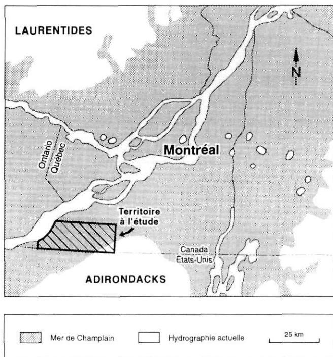
FIGURE 1. Localisation de la zone à l'étude. Limite maximale champlainienne d'après Occhietti, 1989.
