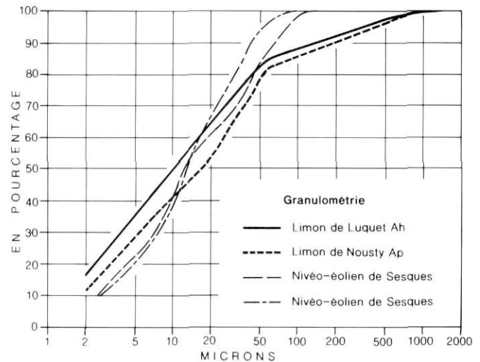
FIGURE 7. Comparaison des courbes granulométriques d'un sédiment nivéo-éolien actuel des Pyrénées et du loess des terrasses de Nousty et Luquet. La seule différence notable réside dans la répartition des 15 % à 18 % de fraction sableuse.
