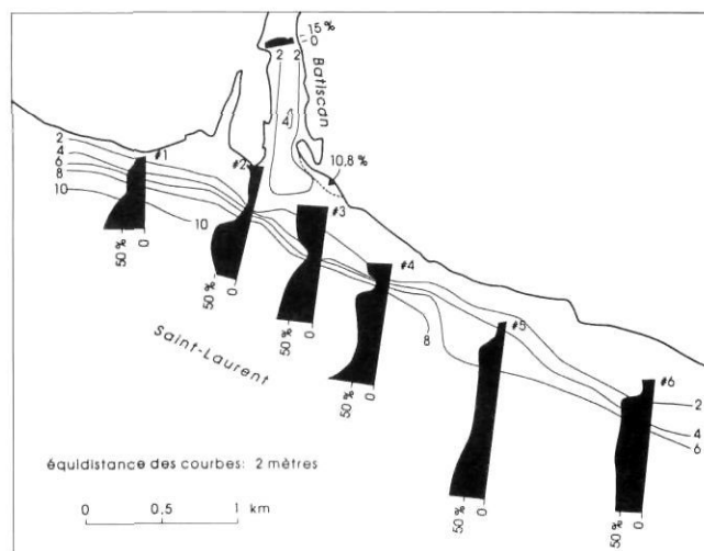
FIGURE 9. Pourcentage brut de minéraux lourds dans les sables très fins (63 à 125 \mu\text{m} ) au confluent Saint-Laurent-Batiscan.
