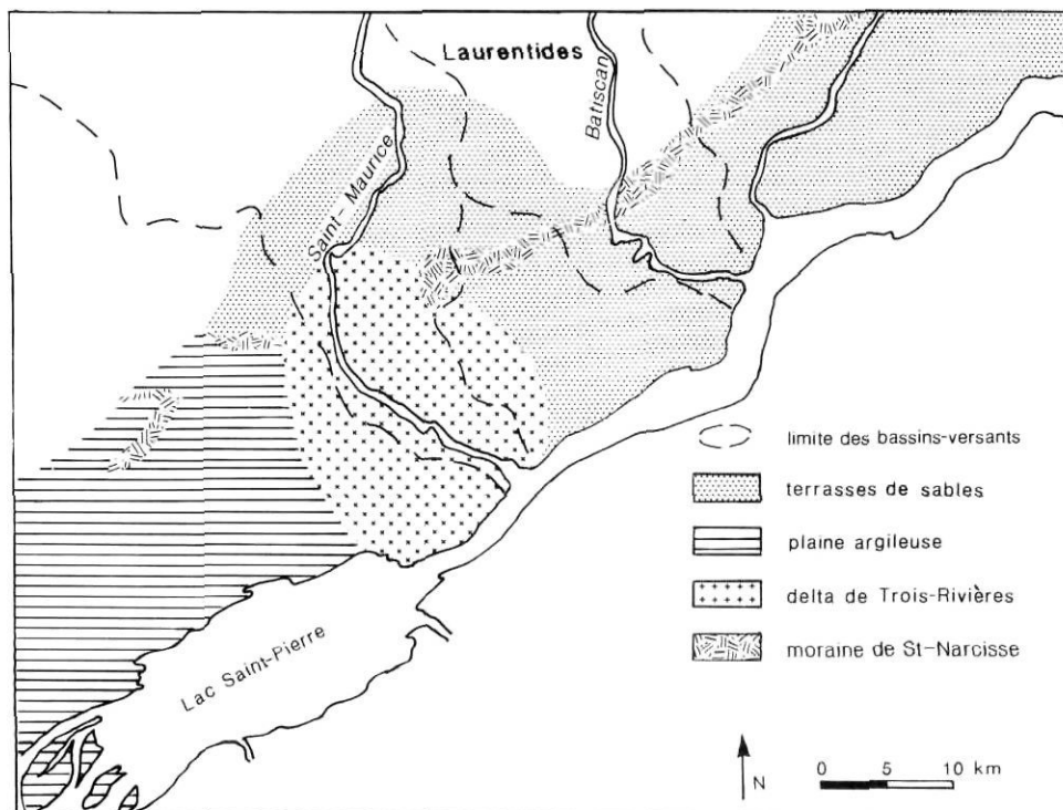
FIGURE 6. Texture du matériel meuble des bassins-versants des rivières Saint-Maurice et Batiscan d'après Gadd (1971).
