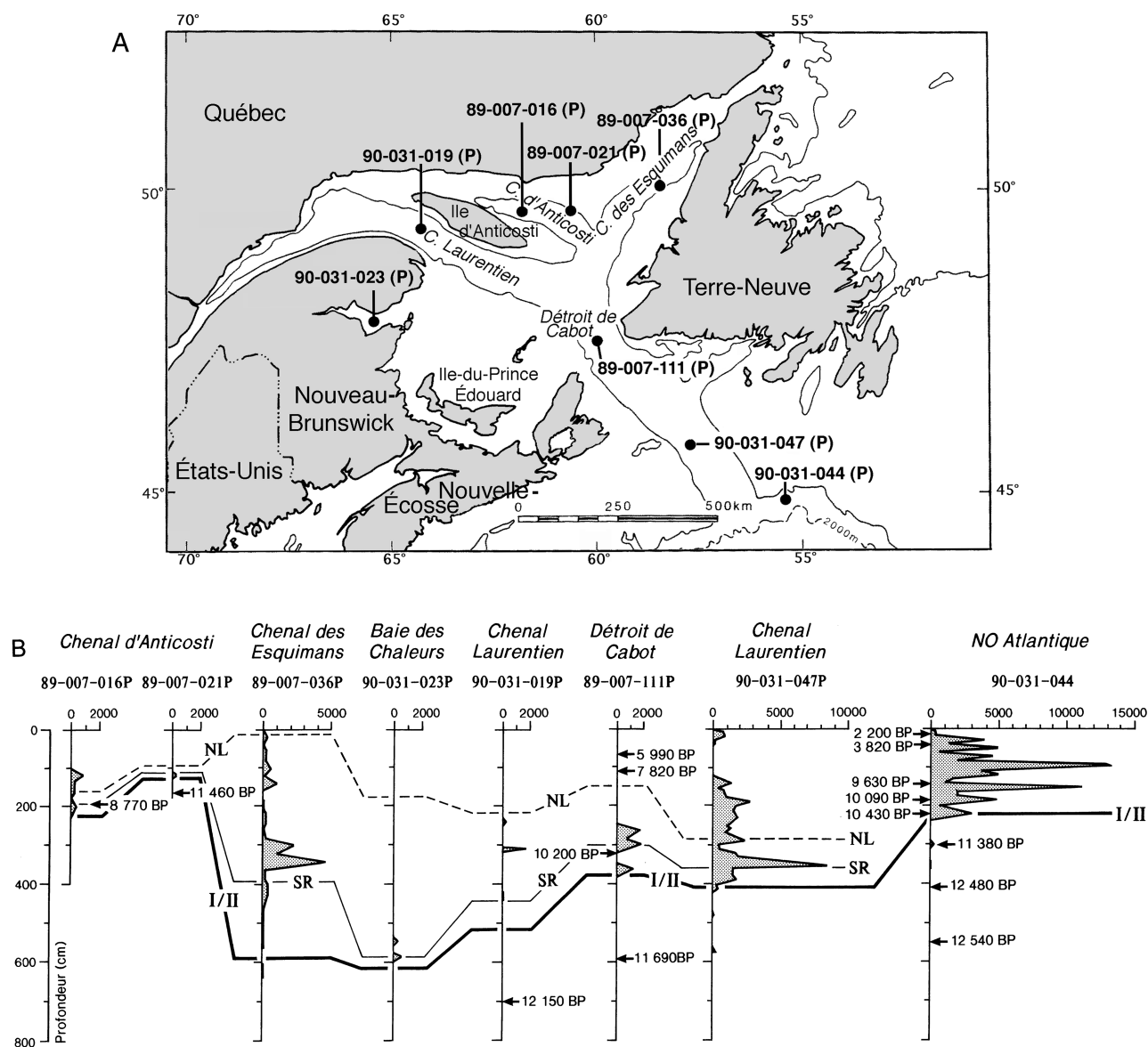
FIGURE 4. Distribution postglaciale des kystes du type Alexandrium excavatum dans le golfe du Saint-Laurent et le chenal Laurentien. Les éléments de stratigraphie et les données palynologiques sont tirées de plusieurs sources (voir les références au tabl. I). A) Localisation des sites de carottage (P = carotte par piston). B) Concentration des kystes du type Alexandrium excavatum (kystes.cm -3 ) par rapport à la profondeur. Les âges au 14 C sont issus de mesures par accélérateur de particules réalisées sur des coquilles de lamellibranches ou sur des tests de foraminifères ; ils sont corrigés de -410 ans afin de tenir compte de la différence entre les réservoirs atmosphériques et océaniques (Rodrigues et al. , 1993 ; de Vernal et al. , 1993, 1996b). Outre les âges au 14 C, quelques repères écostratigraphiques faisant référence aux grandes zones d'assemblages de dinokystes sont utilisés à des fins de corrélations régionales (I/II = transition de l'écozone I à l'écozone II marquée par le passage de population à Péridiniales à des populations à Gonyaulacales ; SR = abondance maximale de Spiniferites ramosus ; NL = abondance maximale de Nematosphaeropsis labyrinthus ; voir de Vernal et al. , 1993).
