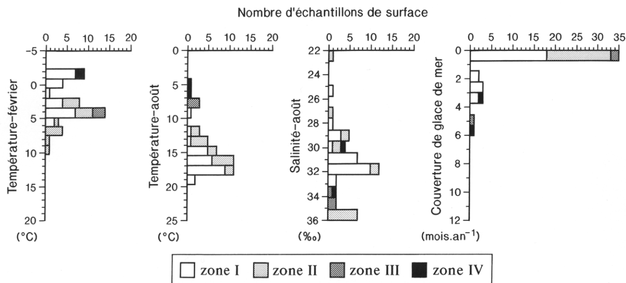
FIGURE 2. Histogramme de fréquence des kystes du type Alexandrium excavatum par rapport aux conditions de surface (les zones I à IV correspondent à celles illustrées sur la fig. 1).
