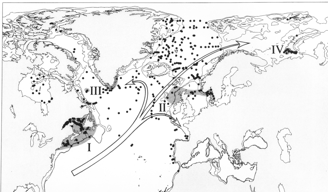
FIGURE 1. Carte de distribution des kystes du type Alexandrium excavatum dans les sédiments récents de l'Atlantique Nord et de ses bassins adjacents. Les sites d'échantillonnage sont indiqués par des points. Les zones tramées I à IV correspondent aux zones caractérisées par la présence de kystes du type Alexandrium excavatum . Les flèches illustrent schématiquement la trajectoire de la dérive nord-atlantique et de ses principales branches, orientale et occidentale.
