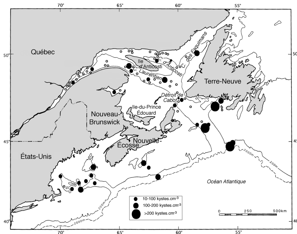
FIGURE 3. Abondance (kystes. \text{cm}^{-3} ) des kystes du type Alexandrium excavatum dans les sédiments de surface de l'estuaire et du golfe du Saint-Laurent et le long des marges continentales dans le domaine atlantique. Tous les sites d'échantillonnage et d'analyse sont reportés sur la figure : les cercles noirs font état des concentrations et les ronds ouverts (o) correspondent aux échantillons dans lesquels le type Alexandrium excavatum n'a pas été observé, ses concentrations étant inférieures aux limites de comptage.
