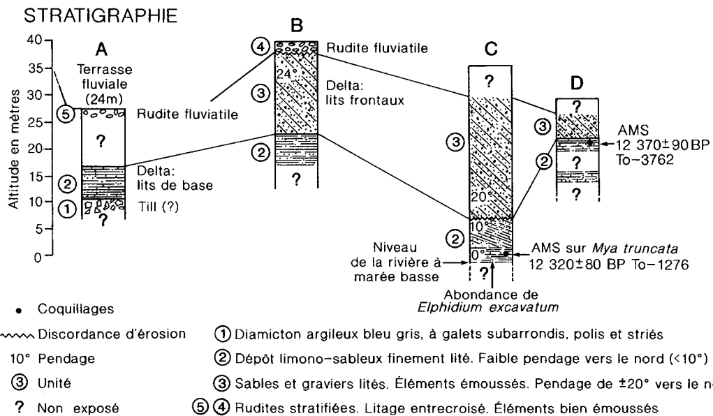
FIGURE 20. Contexte géomorphologique et stratigraphique du delta de contact glaciaire de la rivière Madeleine.
