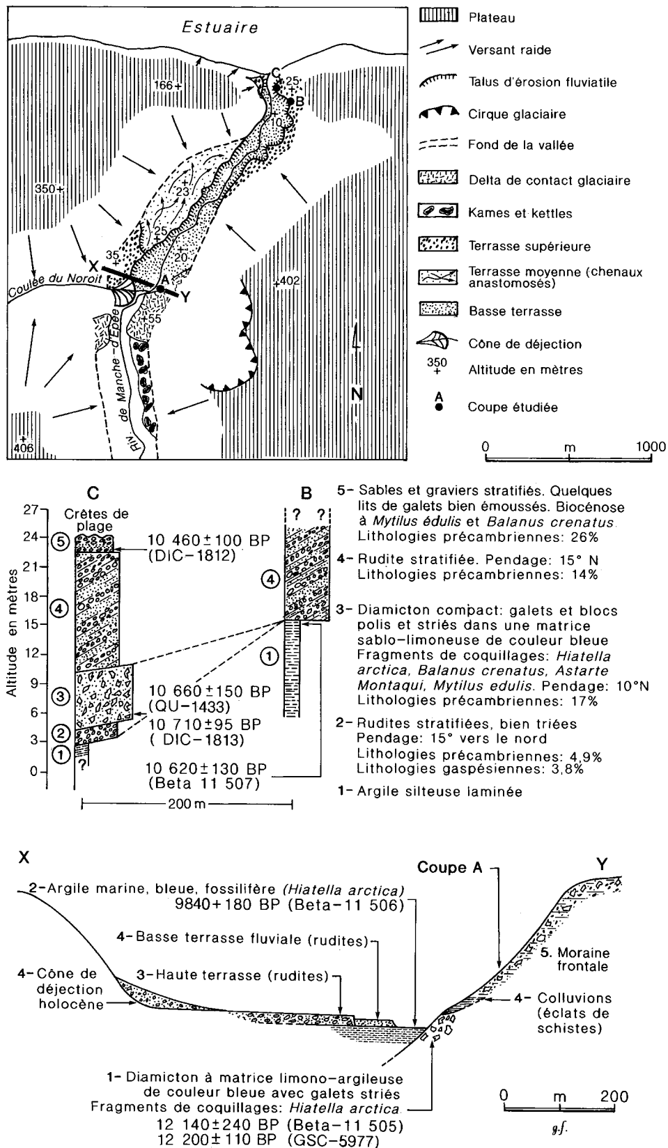
FIGURE 17. Géomorphologie et stratigraphie des dépôts meubles près de l'embouchure de la vallée du ruisseau de Manche d'Épée.
