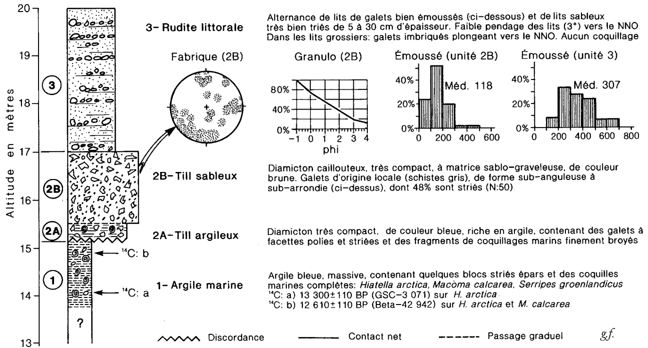
FIGURE 4. Stratigraphie de la coupe de l'anse au Naufrage (localisation à la figure 3). Stratigraphy of exposure at Anse au Naufrage (see Fig. 3 for location).
