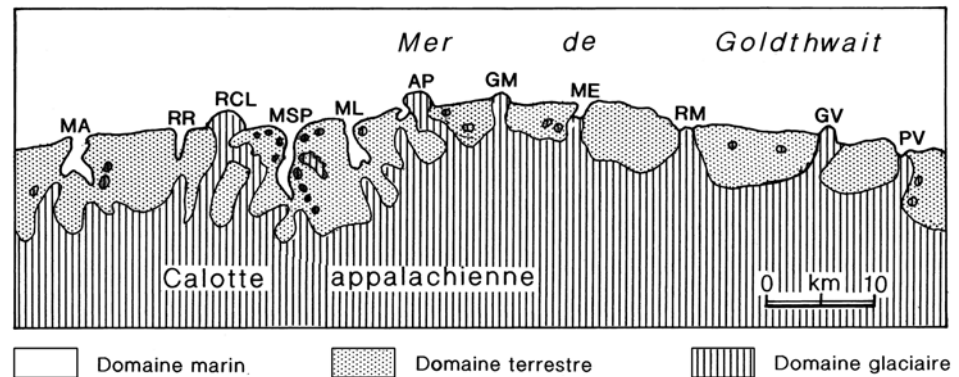
FIGURE 28. L'étendue proposée pour le couvert glaciaire dans le nord de la Gaspésie durant le Dryas ancien. Voir la figure 23 pour les abréviations.
