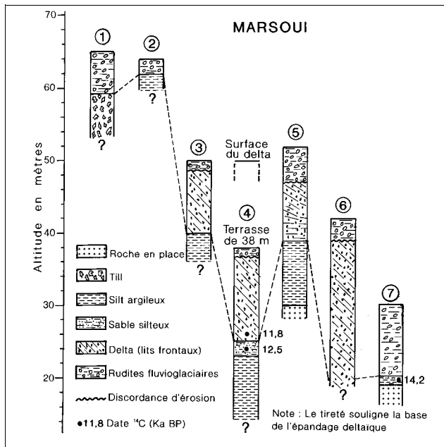
FIGURE 5. Stratigraphie des terrasses de la vallée de Marsoui. Le tireté souligne la base de l'épandage fluvio-glaciaire qui devient deltaïque à la confluence des deux vallées (rivières Marsoui et Marsoui Est). La localisation des coupes est indiquée à la figure 3.
