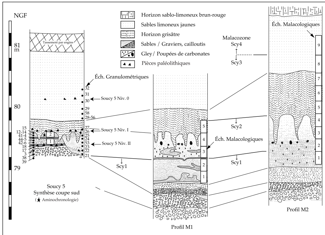
FIGURE 9. Levés stratigraphiques de la coupe sud du gisement de Soucy 5 et des profils M1 et M2. Localisation des échantillons granulométriques et malacologiques.
