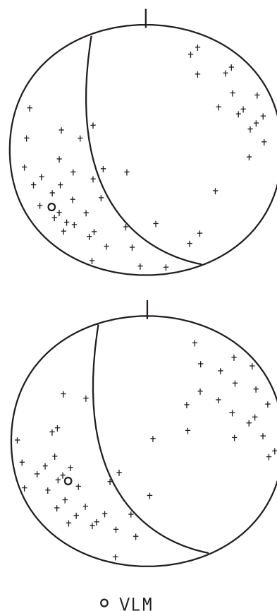
FIGURE 13. Deux stéréogrammes de Schmidt représentant l'orientation et l'inclinaison du grand axe des éléments de deux cônes apicaux (hémisphère inférieure). L'arc de cercle représente la surface du cône apical (1 : pente : 42°; 2 : pente : 45°). VLM : vecteur linéaire moyen.
