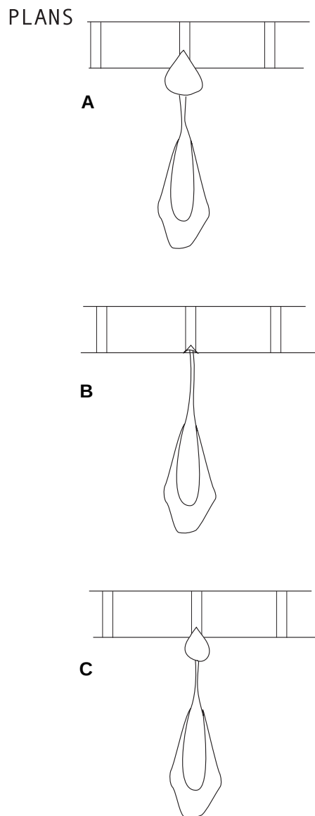
FIGURE 12. Évolution des profils des modelés de coulées de débris : A) cône apical constitué ; B) cône apical purgé ; C) cône apical en cours de constitution.
