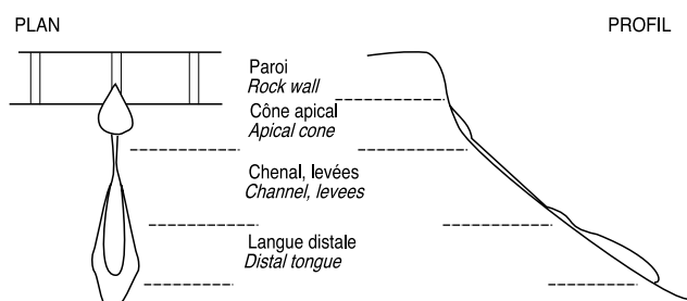
FIGURE 6. Cône apical et modelés édifiés par une coulée de débris. Apical cone and landforms built by a debris flow.
