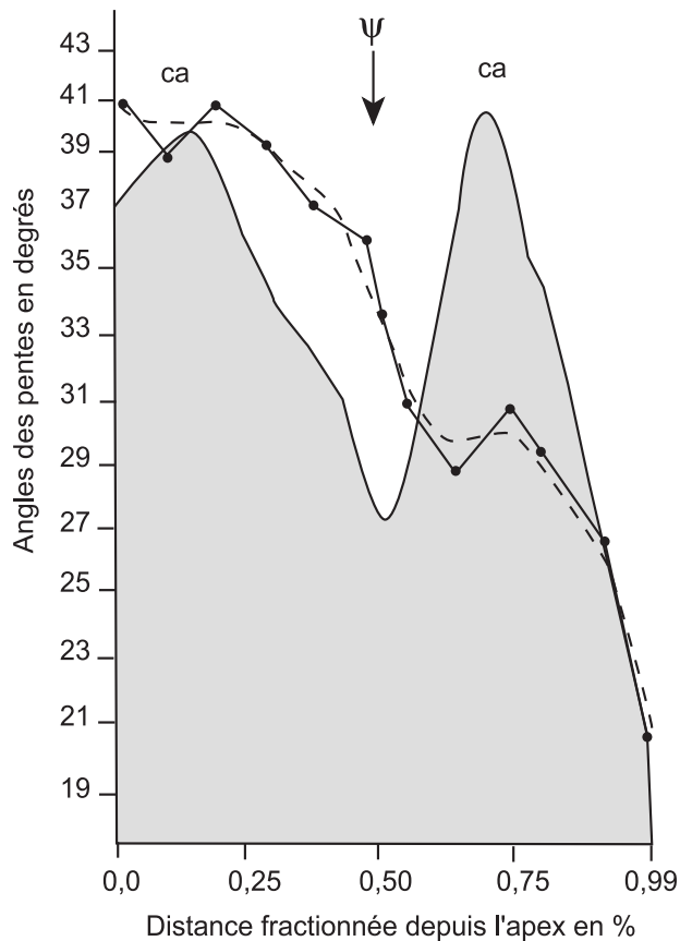
FIGURE 9. Exemple de profil d'éboulis. Abscisse : distance fractionnée depuis l'apex ; ordonnée : valeur des angles ; ligne pleine et point : segment et interpolation linéaire ; trait continu : pente ; trait discontinu : approximation Spline cubique ; grisé : dérivée seconde de l'approximation de la Spline cubique ; flèche et \psi : point de rupture ; ca : concavité.
