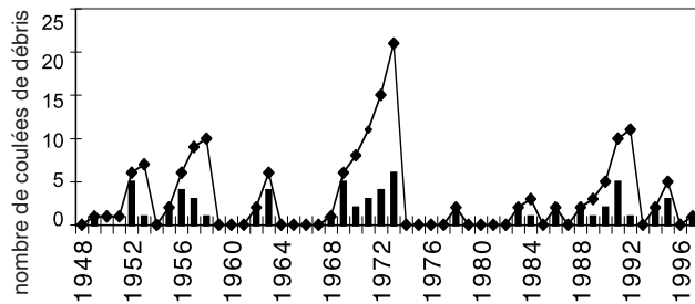
FIGURE 15. Chronologie des coulées de débris de versants du plateau de Bure entre 1948 et 1997. La courbe met en évidence la succession de cycles de déclenchement des coulées ; elle représente des événements cumulés entre des phases de repos.
